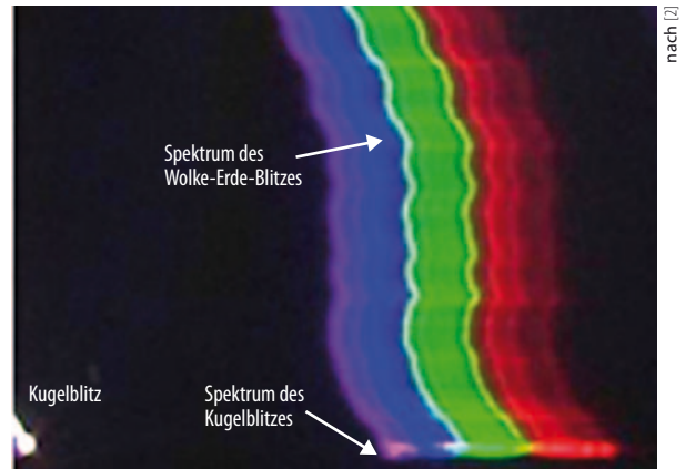
Das erste Bild der Videokamera zeigt die Erzeugung des Kugelblitzes (unten links). Das dazugehörige Spektrum ist unterhalb des Spektrums des Blitzes als schmaler Streifen zu erkennen.
